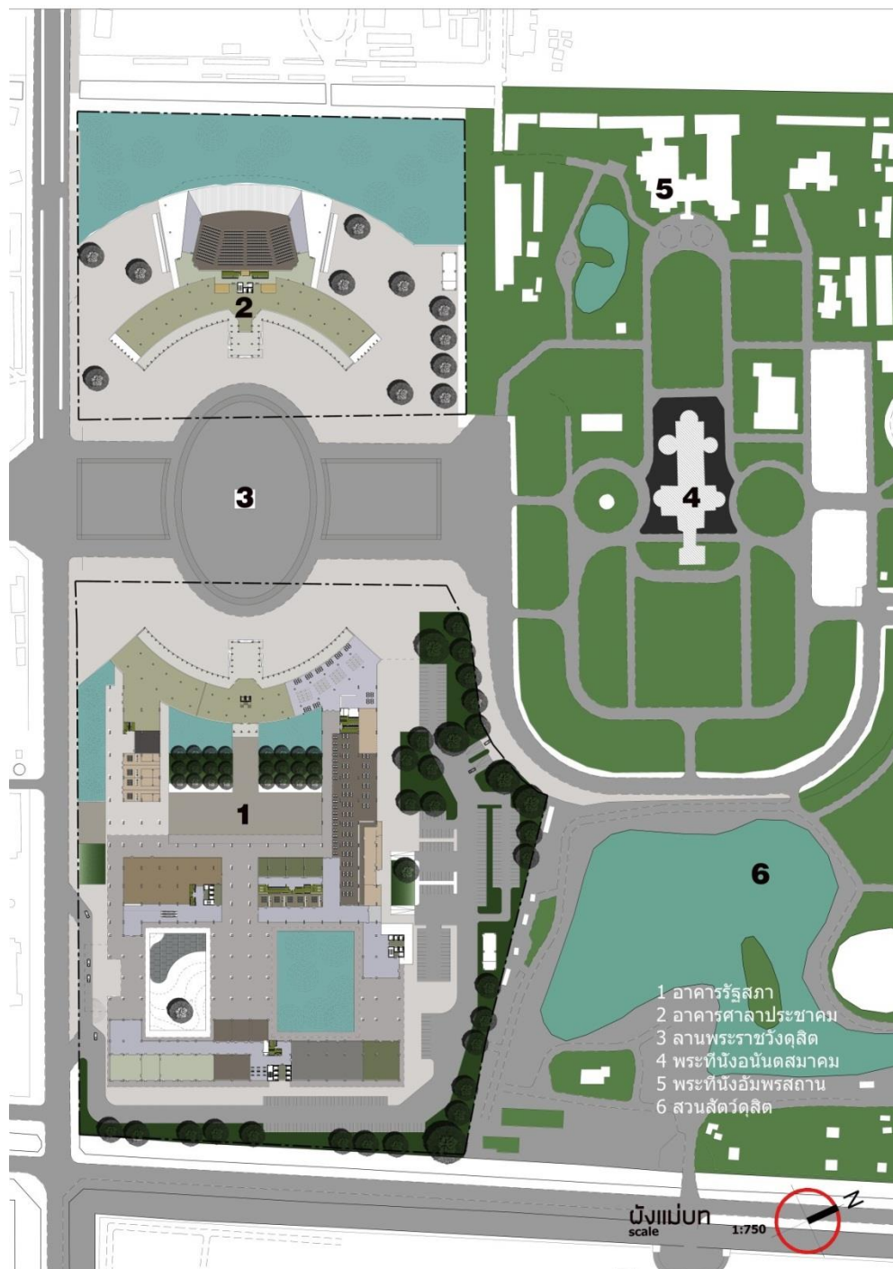
ภาพที่ 80 ผังแม่บทโครงการรัฐสภาแห่งใหม่
