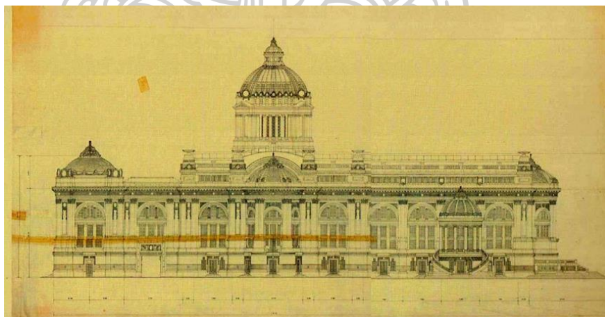
ภาพที่ 116 แบบของพระที่นั่งอนันตสมาคม ที่มา สำนักพิมพ์ Lizem
