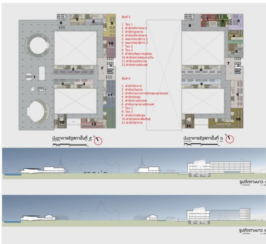
ภาพที่ 86 ผังพื้นที่ 3-6 อาคารรัฐสภา
