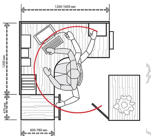
ภาพที่ 51 ขนาดมิติของการจัดโต๊ะทำงาน
