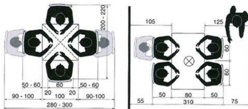
ภาพที่ 49 ขนาดมิติของการจัดโต๊ะและเก้าอี้ห้องประชุม
