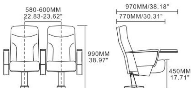
ภาพที่ 47 ขนาดมิติของเก้าอี้ห้องประชุม
