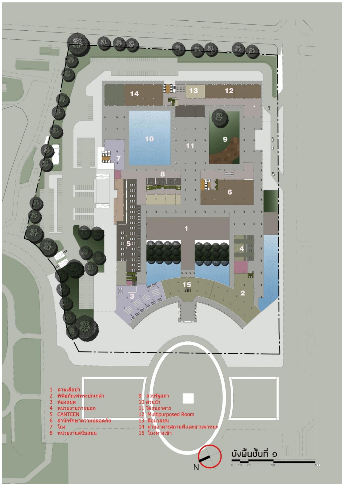
ภาพที่ 82 ผังพื้นที่ชั้นที่ 1 อาคารรัฐสภา
