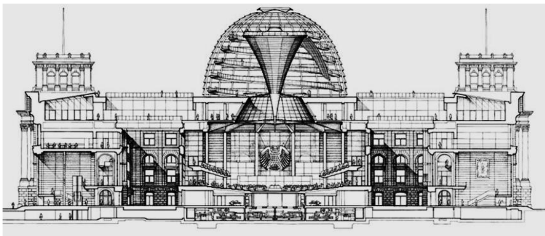
ภาพที่ 29 รูปตัดด้านขวางที่แสดงให้เห็นความสัมพันธ์ของ Dome และ Chamber ที่มา Ga Document Extra 12
