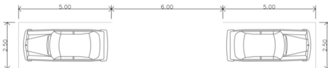
ภาพที่ 52 ขนาดมิติของการจัดที่จอดรถ
