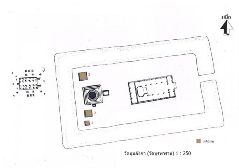
ภาพที่ 41 แผนผังเจดีย์รายวัดมumlลงกา (วัดบูรพาราม)
