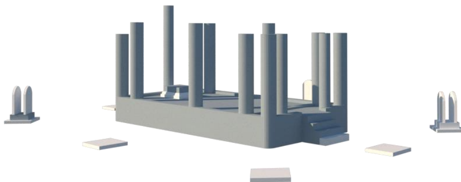
ภาพที่ 143 ภาพ 3 มิติสภาพปัจจุบัน โบสถ์วัดมุลังกา (วัดบูรพาราม)
