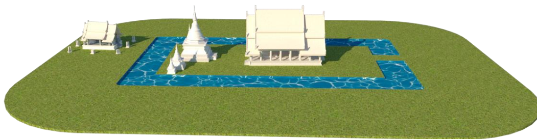
ภาพที่ 153 ภาพสันนิษฐาน 3 มิติวัดมumlลंगा (วัดบูรพาราม) ด้านทิศใต้
