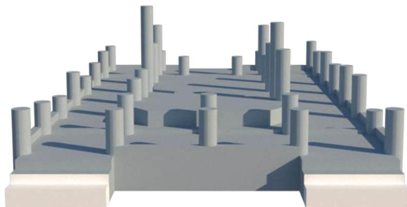
ภาพที่ 139 ภาพ 3 มิติสภาพปัจจุบันวิหารวัดมumlลंगा (วัดบูรพาราม)
